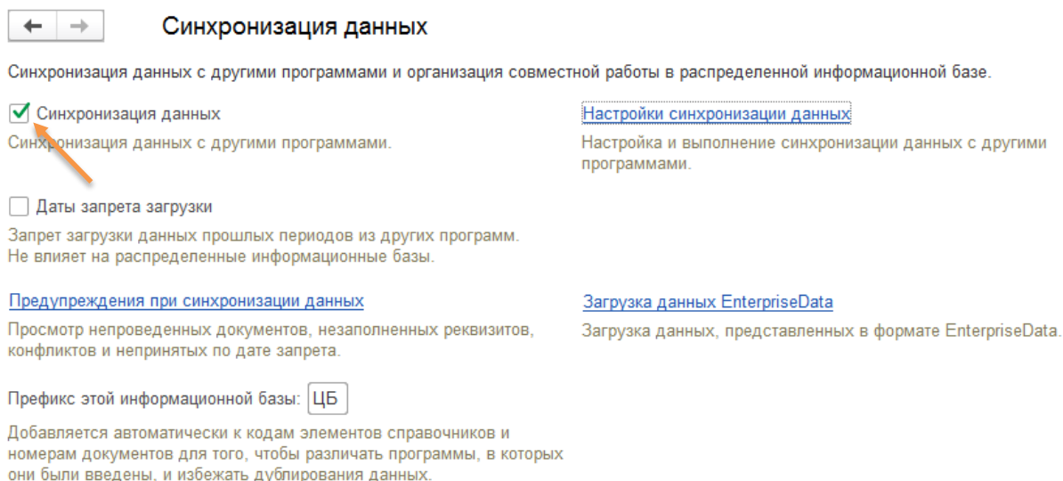
Рисунок 5. Синхронизация данных
